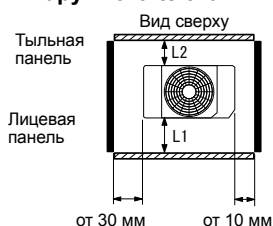
Рис. 2 Установка одного наружного блока
