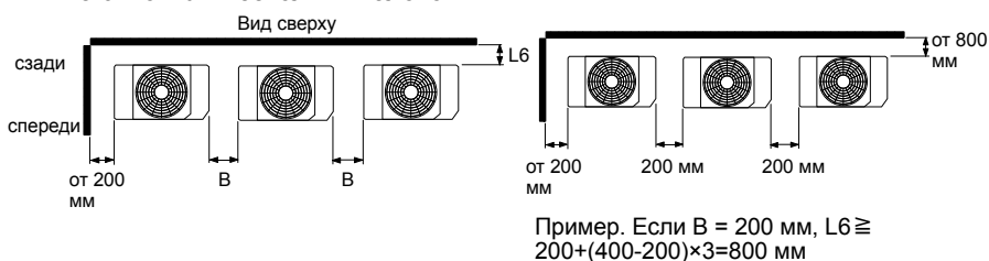
Рис.9 Монтаж нескольких блоков
