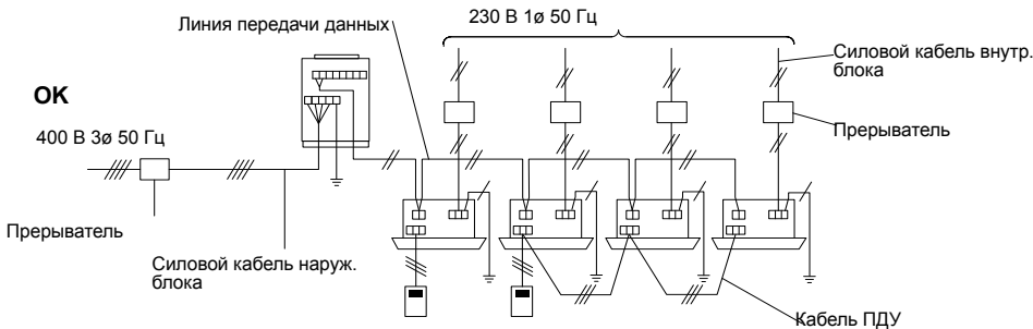
Рис. При подключении одного наружного блока (прерыватели)
