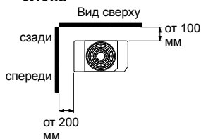
Рис. 8 Монтаж одного блока
