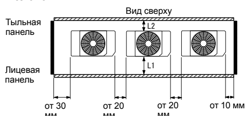
Рис. 3 Установка нескольких наружных блоков
