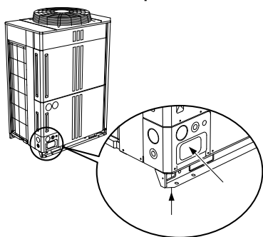
Рис. А Расположение выбиваемого отверстия
